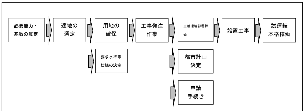
図 2-2-11 仮設焼却炉等の設置フロー
