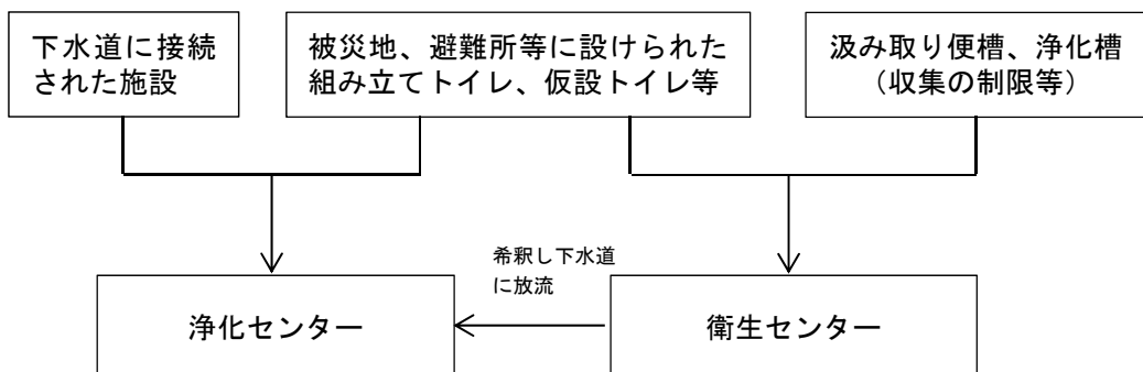
図 2-2-3 災害時のし尿の処理フロー
