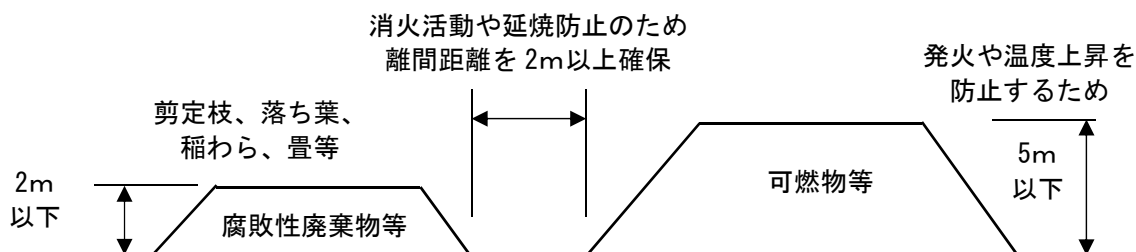
図 2-2-10 理想的な仮置場の廃棄物堆積状況
