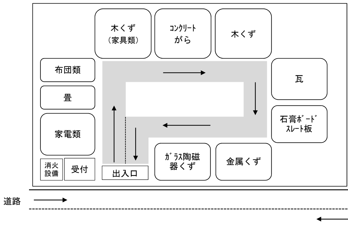
図 2-2-8 仮置場の分別配置図の例
