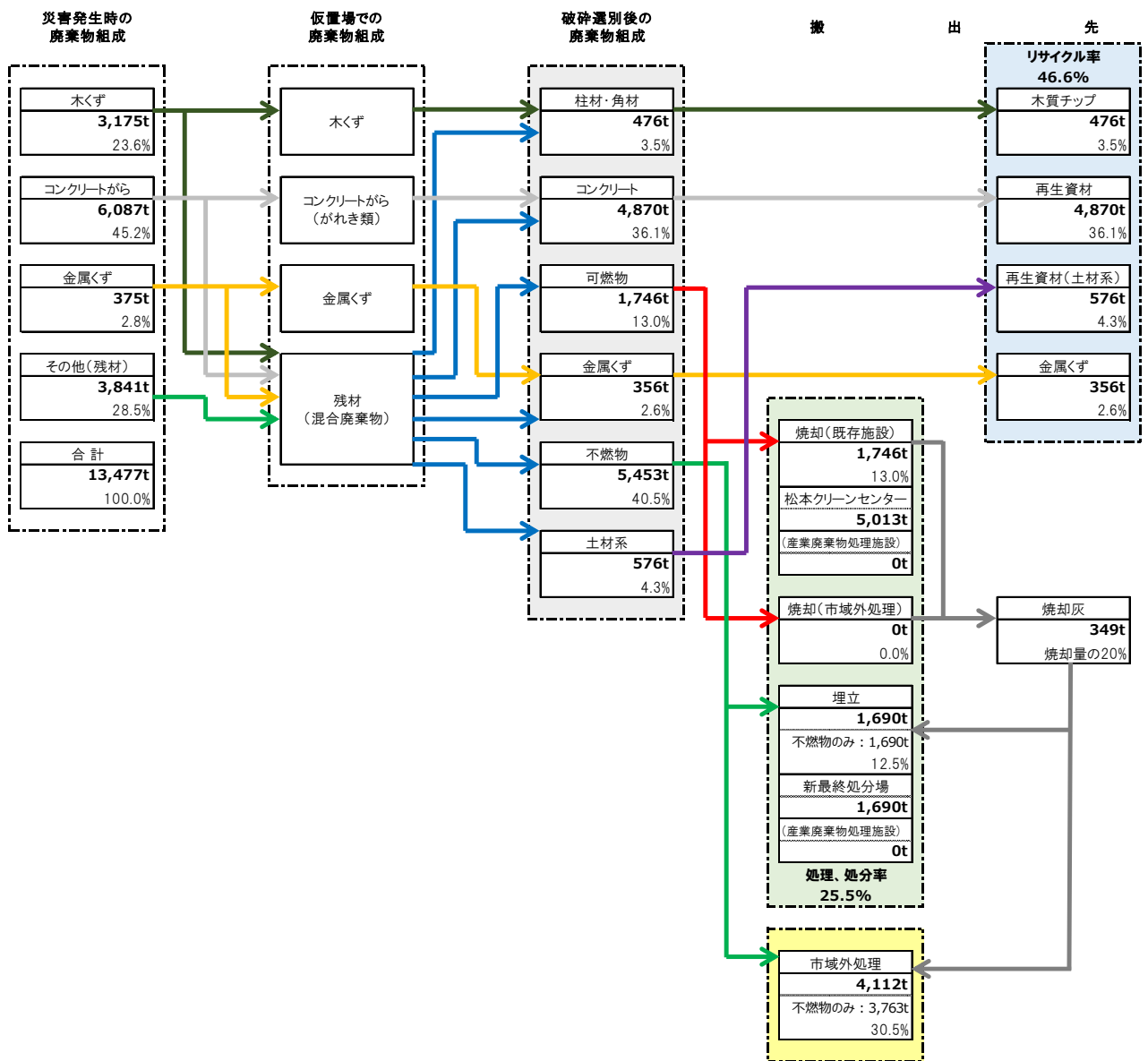
図2-2-4 糸魚川ー静岡構造線断層帯（全体）の地震における災害廃棄物処理フロー
