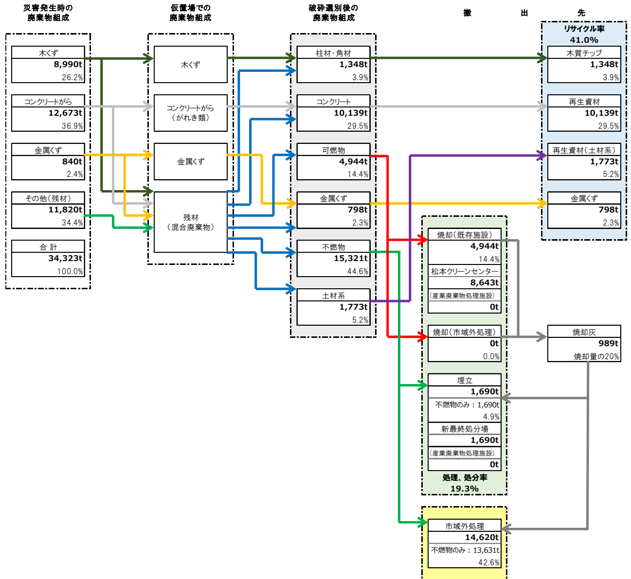
図 2-2-5 境峠・神谷断層帯（主部）の地震における災害廃棄物処理フロー
