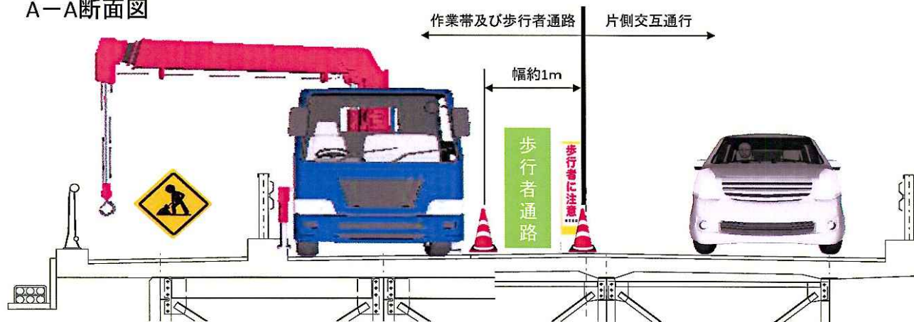
A-A断面図
