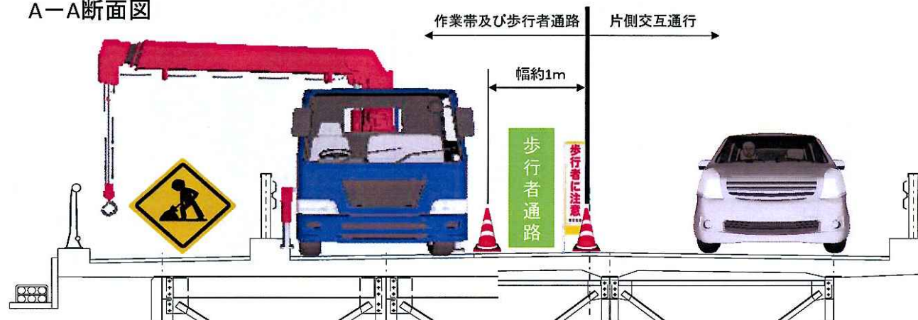
A-A断面図
