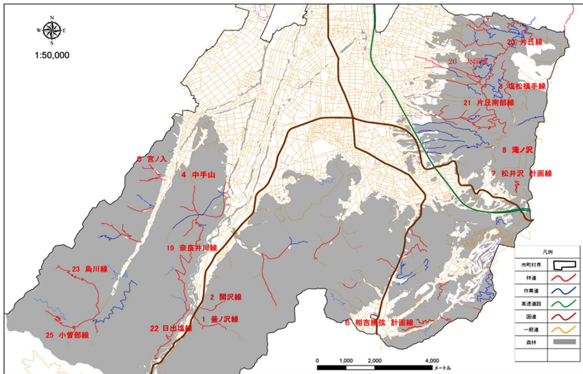
塩尻市 路網整備計画図(1/2)
