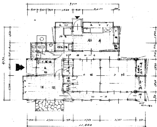
1階平面図 S.1:100.
