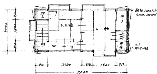
2階平面図 S.1:100.
