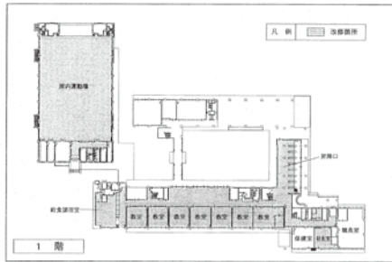
塩尻中学校 塩尻中学校大規模改修工事（平面図）
